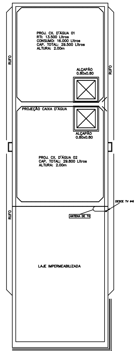
COB.CAIXA D'AGUA ESCALA 1:100
