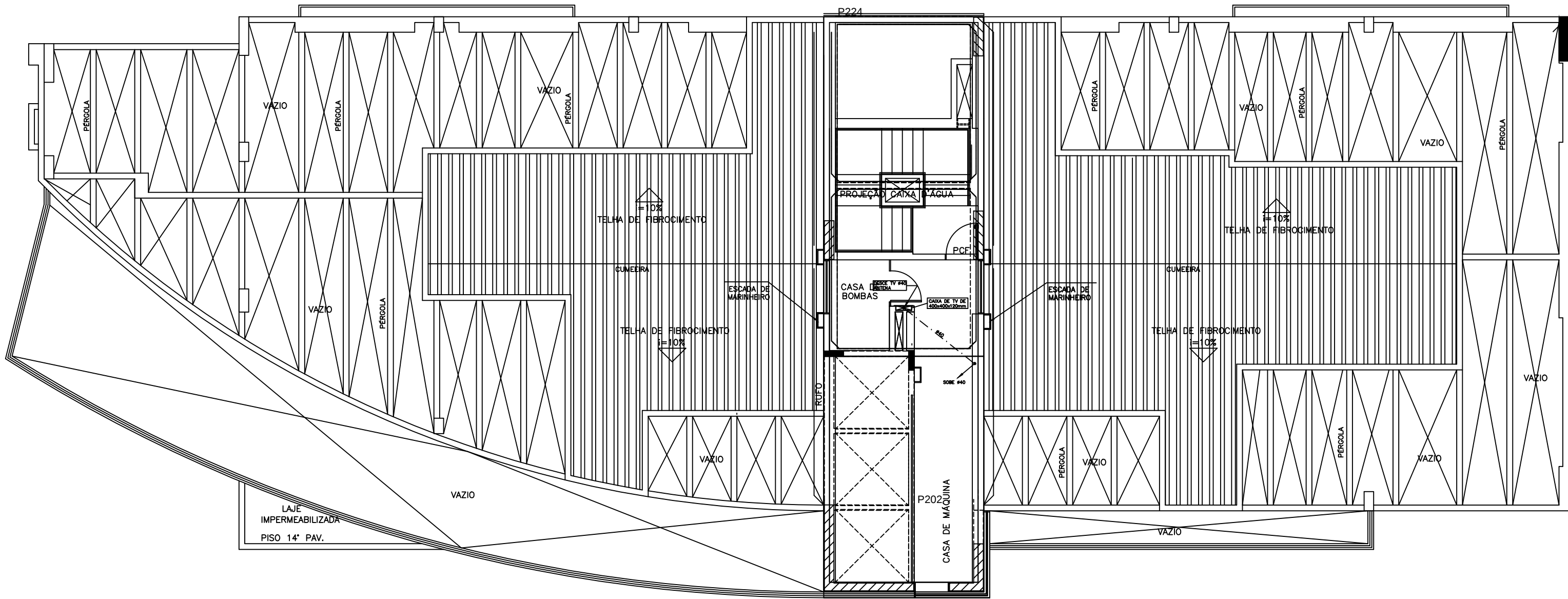
PLANTA BAIXA COBERTURA – BLOCO "C" RESIDENCIAL ESCALA 1:50
